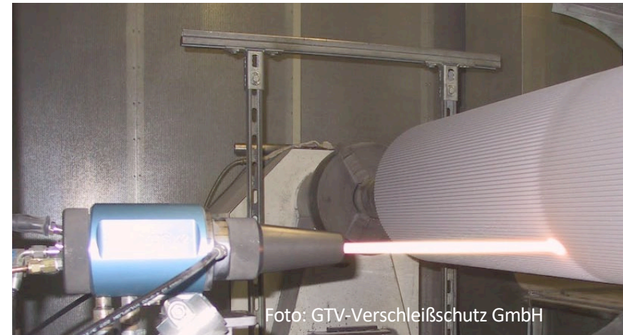
Pulverización de polvo con pistola de gas a alta velocidad (HVOF/HVAF): Material
