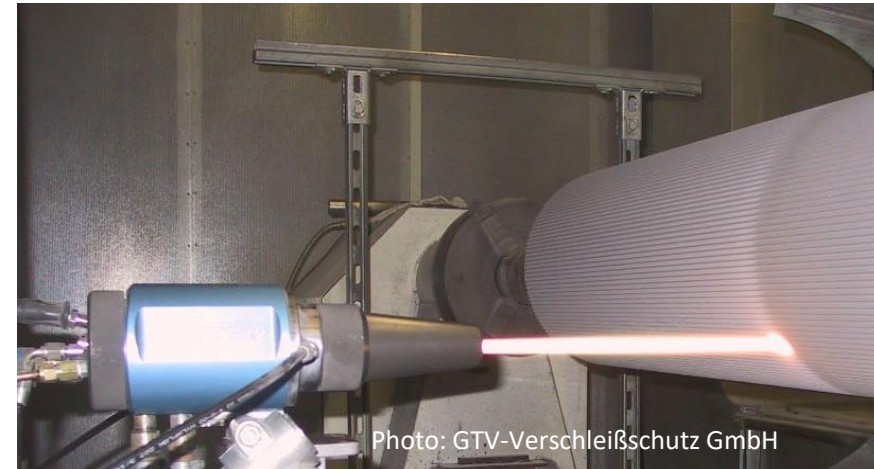
Projection de poudres à la flamme à grande vitesse (HVOF/HVAF): Equipement
