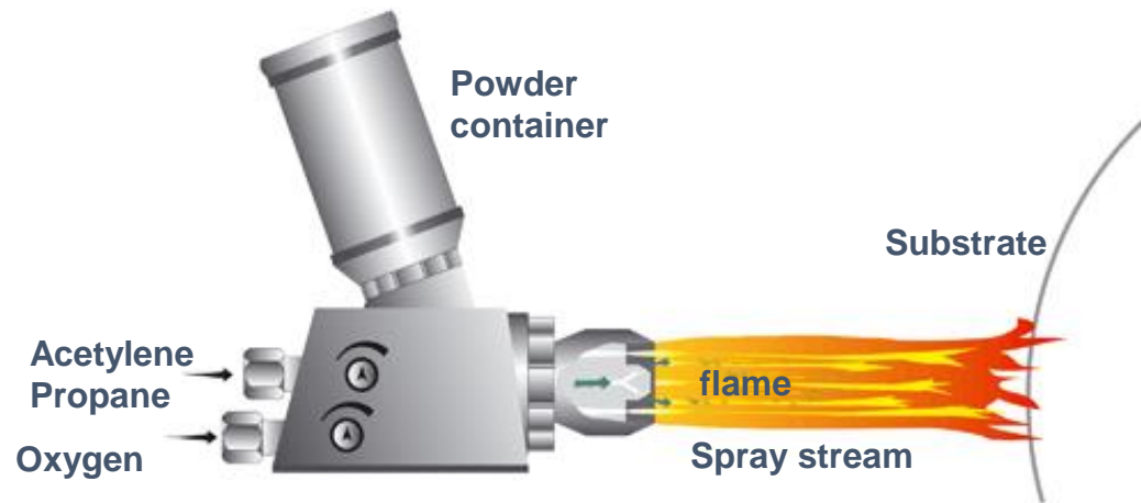
Projection de poudres à la flamme (PFS): Technique
